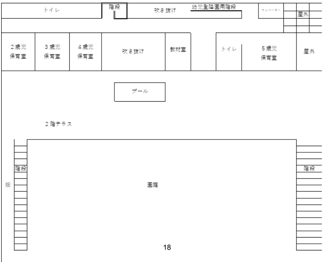
【2階】
