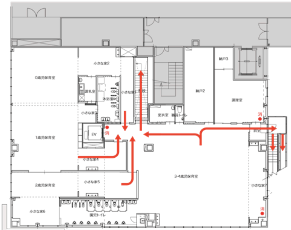
■2階平面図
