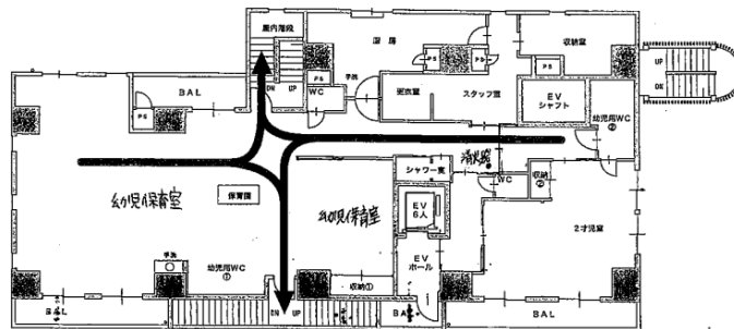
2階見取り図
